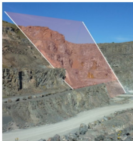
Plan de faille (en rouge) et abattage (front 5)
