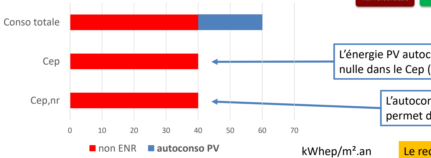
exemple du photovoltaïque
