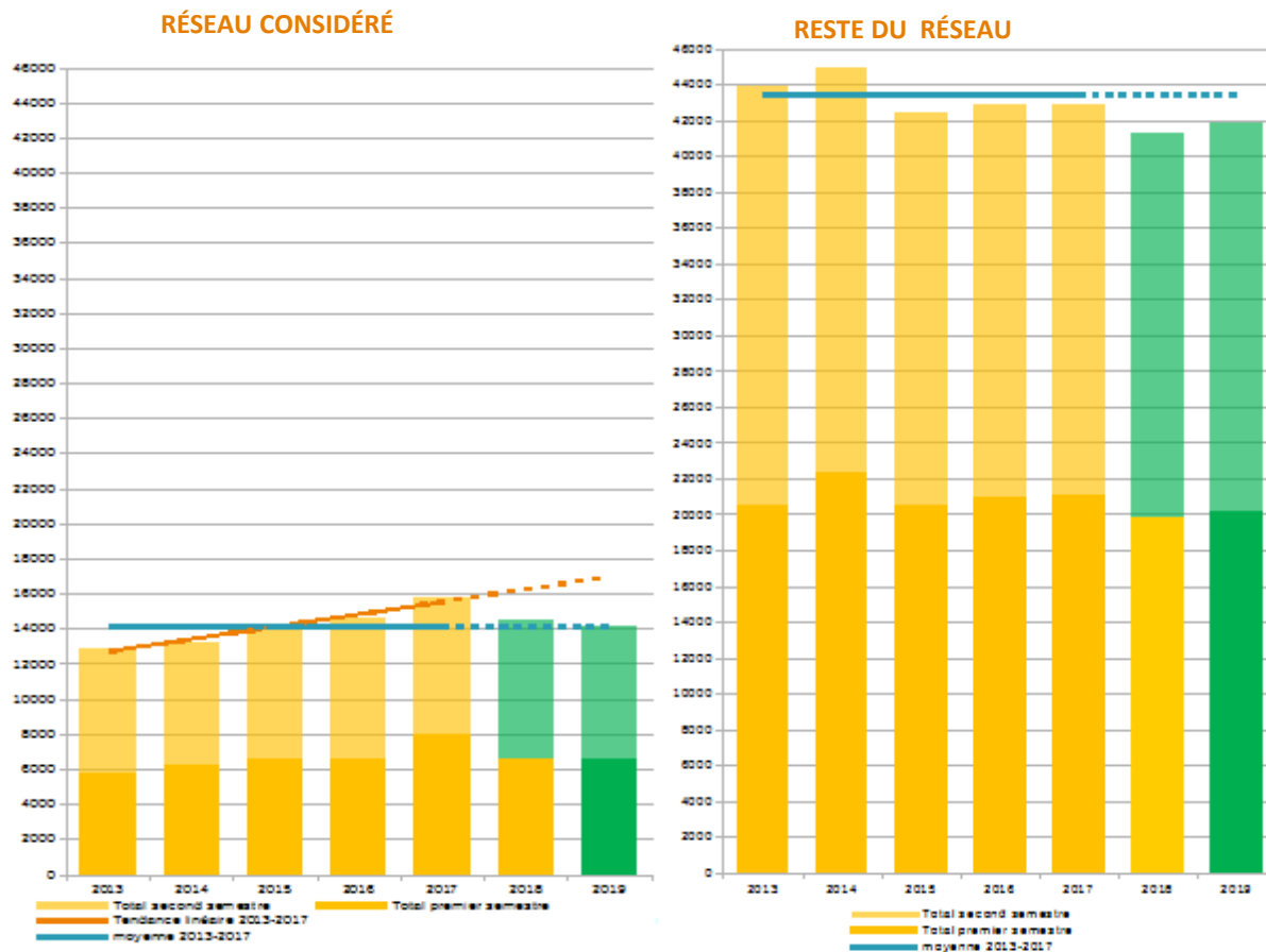
Comparaison du nombre d'accidents sur le réseau considéré et sur le reste du réseau, par année (Sources : BAAC officiel)
