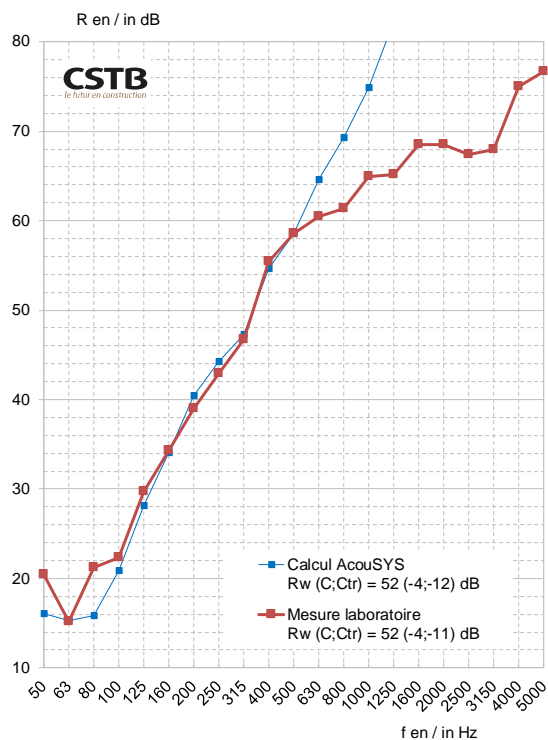
Figure 4-19 : Comparaison calcul/mesure de l'indice d'affaiblissement acoustique R simulé et mesuré sur la toiture avec isolant biosourcé.
