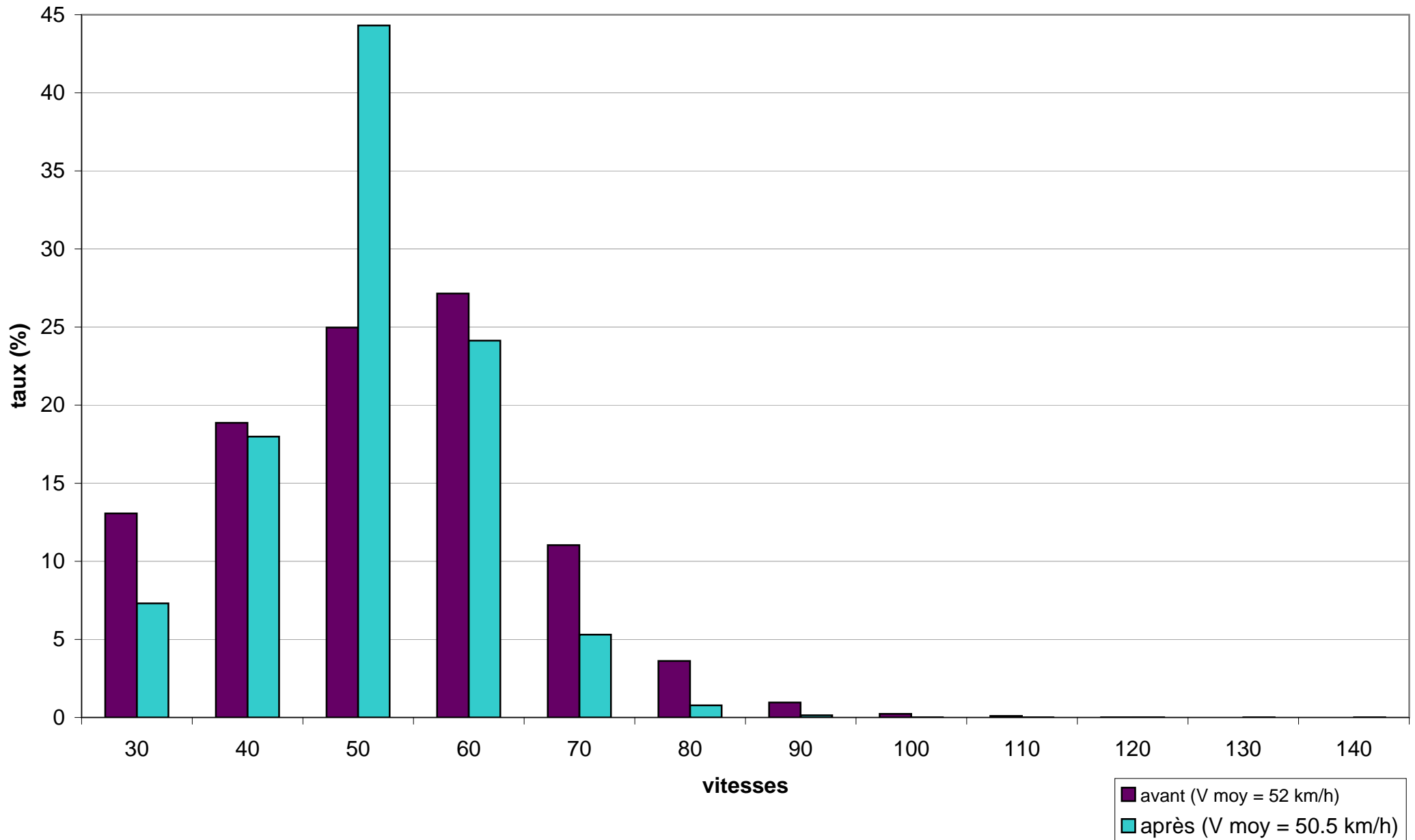
Flavin sens Pont de Salars-Rodez (carrefour RD 911-RD62) comparatif des vitesses avant/après la pose de feux asservis à la vitesse
