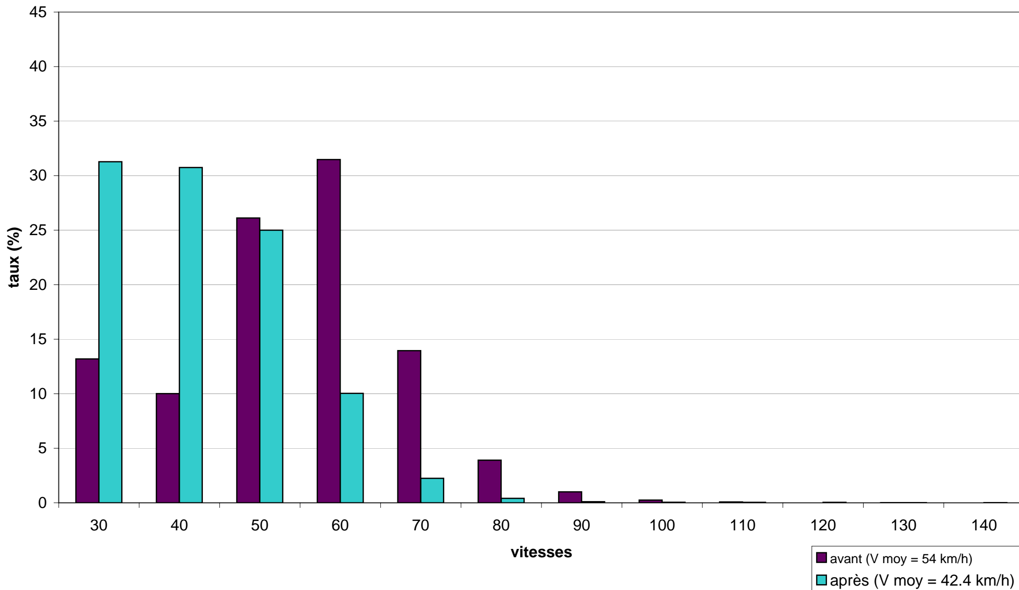
Flavin sens Rodez-Pont de Salars (carrefour RD 911-RD62) comparatif des vitesses avant/après la pose de feux asservis à la vitesse
